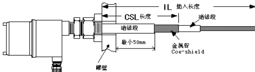
图 1.1 传感器结构图
