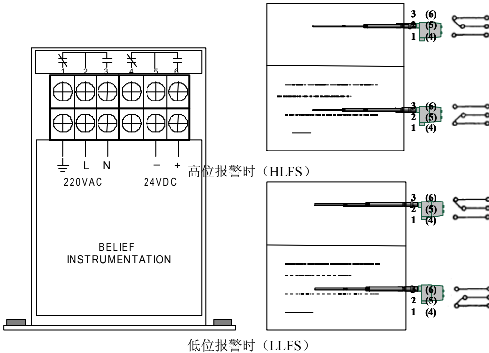
图 4.6 电源及继电器接线图
