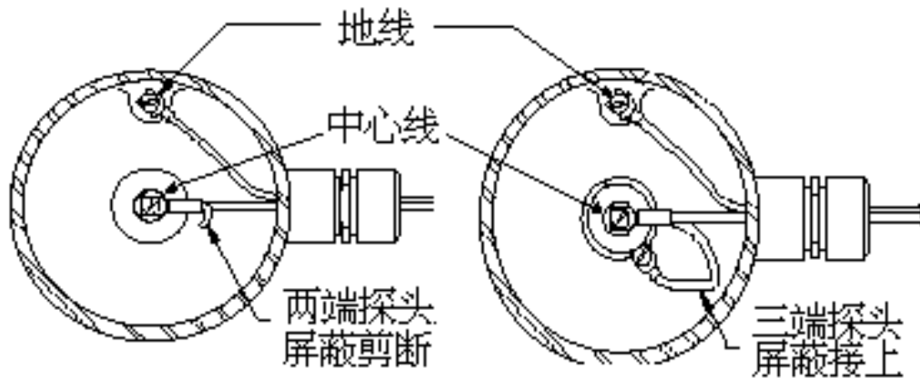
图 4.4 整体接线图
