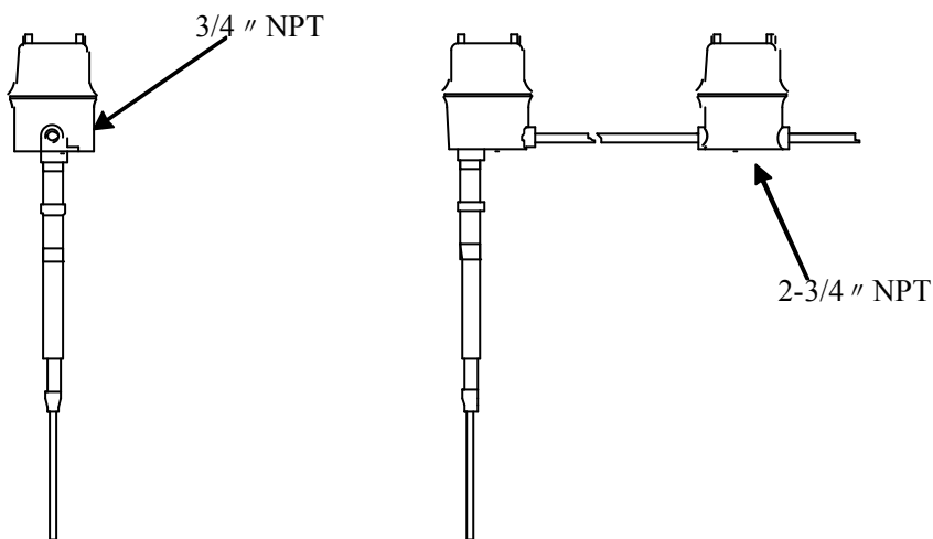
图 4.1 整体型系统安装
