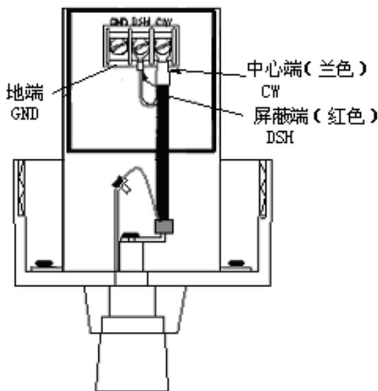
图 4.5 分体接线图
